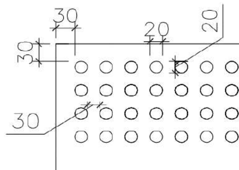
Lochung rund Ø 20 mm
