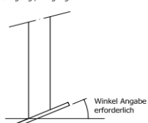
Rohrpfosten mit Fussplatte in Steigung / Neigung
