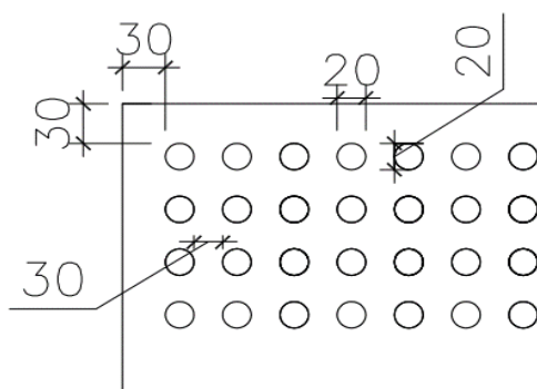
Lochung rund \varnothing 20 mm
