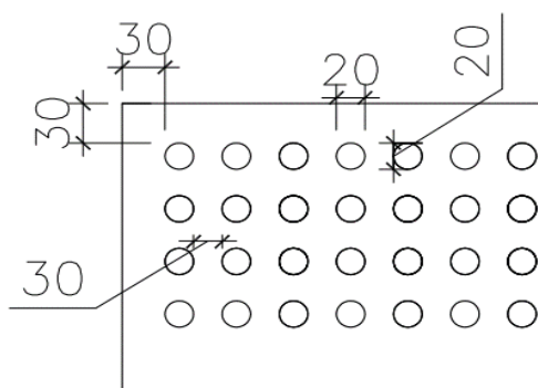
Lochung rund Ø 20 mm
