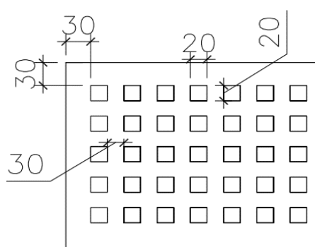
Lochung eckig 20 x 20 mm
